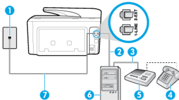
그림 5-13 프린터의 뒷 부분
